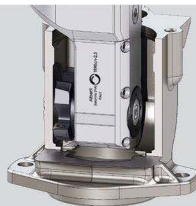
Testa rinvia per spazi ristretti Offset head for reduced spaces
