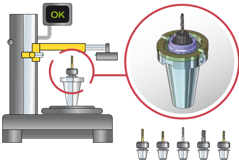
Adattatore per pre-set ISO 50 - Smart Change Tool pot adapters ISO 50 - Smart Change
